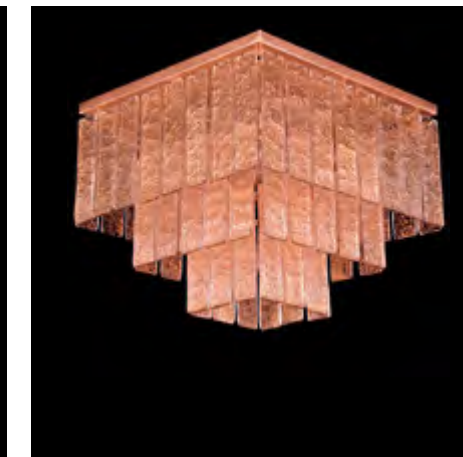
PL7500Q-50x40-U1 W 50 cm - H 40 cm - D 50 cm E14 x 7 20 KG
