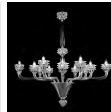
LE0355-6+6-C Ø 105 cm - H 105 cm - C 30 cm - R 14 cm E14 12 x MAX 60W 16 KG
