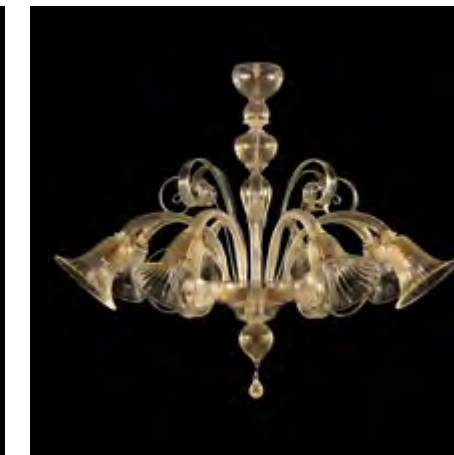
L0560-8-K Ø 100 cm - H 90 cm - C 30 cm - R 12 cm E14 8 x MAX 40W 14 KG
