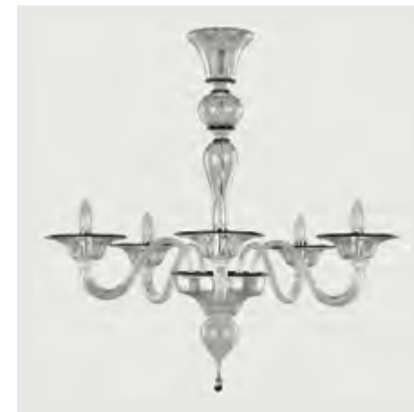
L0360-5-CJ Ø 75 cm - H 80 cm - C 30 cm - R 12 cm E14 5 x MAX 60W 6 KG
