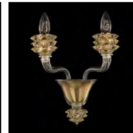
AP0355-2-CK W 25 cm - H 35 cm - D 25 cm E14 2 x MAX 60W 2 KG
