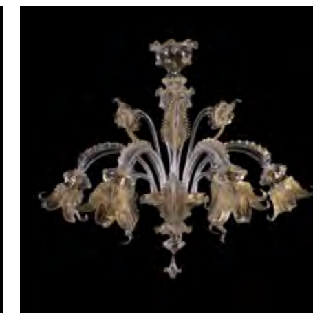
L0086-6-CK Ø 80 cm - H 80 cm - C 30 cm - R 12 cm E14 6 x MAX 40W 13 KG
